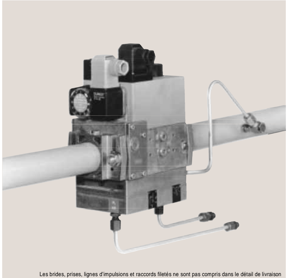
Les brides, prises, lignes d'impulsions et raccords filetés ne sont pas compris dans le détail de livraison
